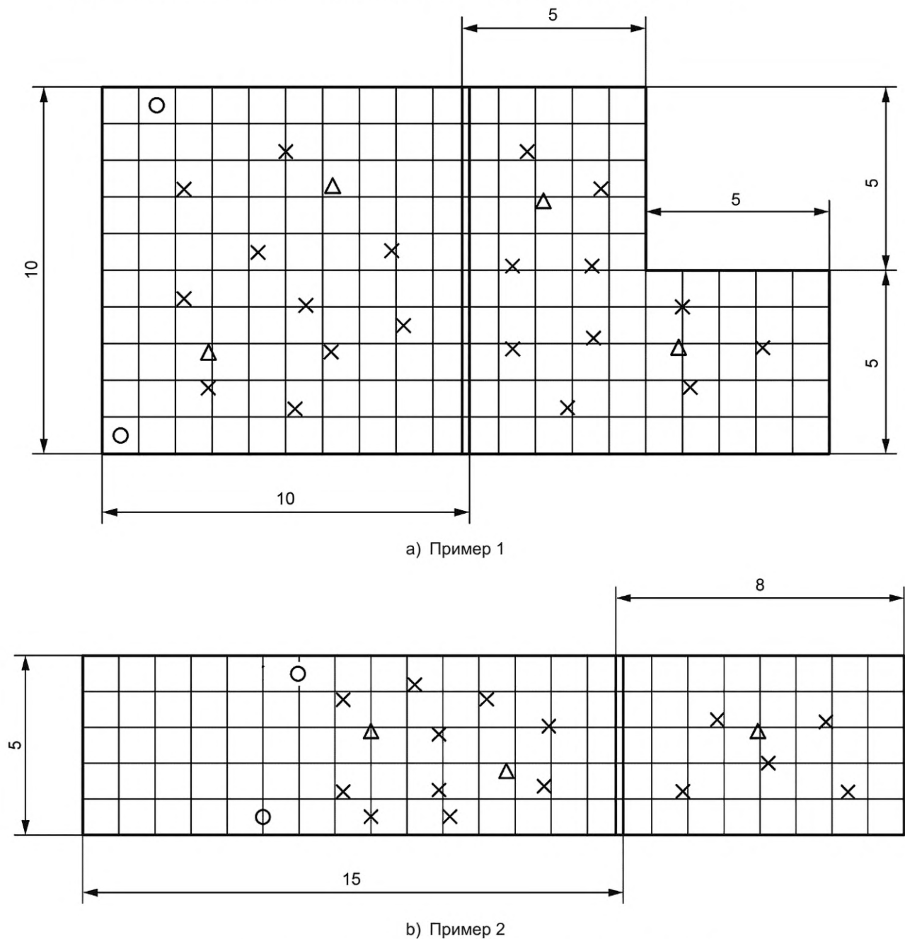
Рисунок D.1 — Горизонтальные измерения, примеры 1—14, лист 1
