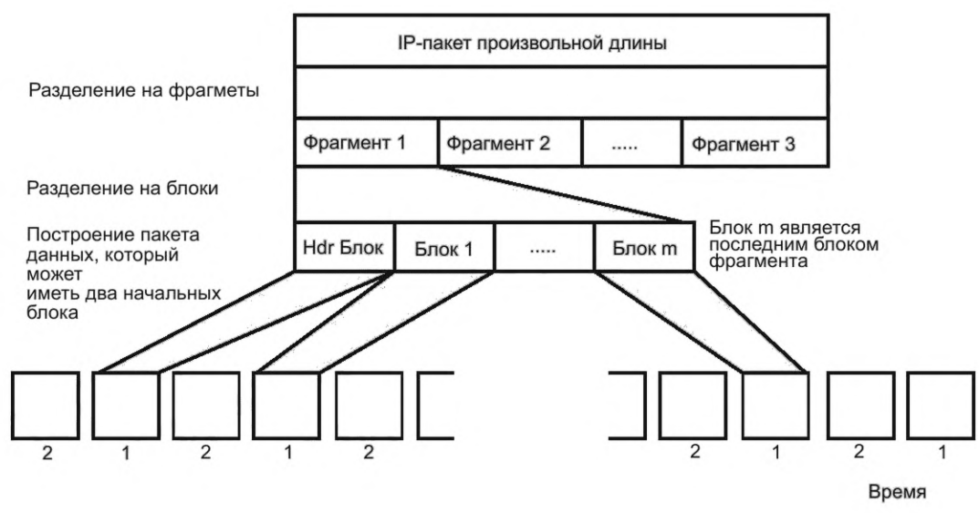
Рисунок 108 — Фрагментация IP-пакета
