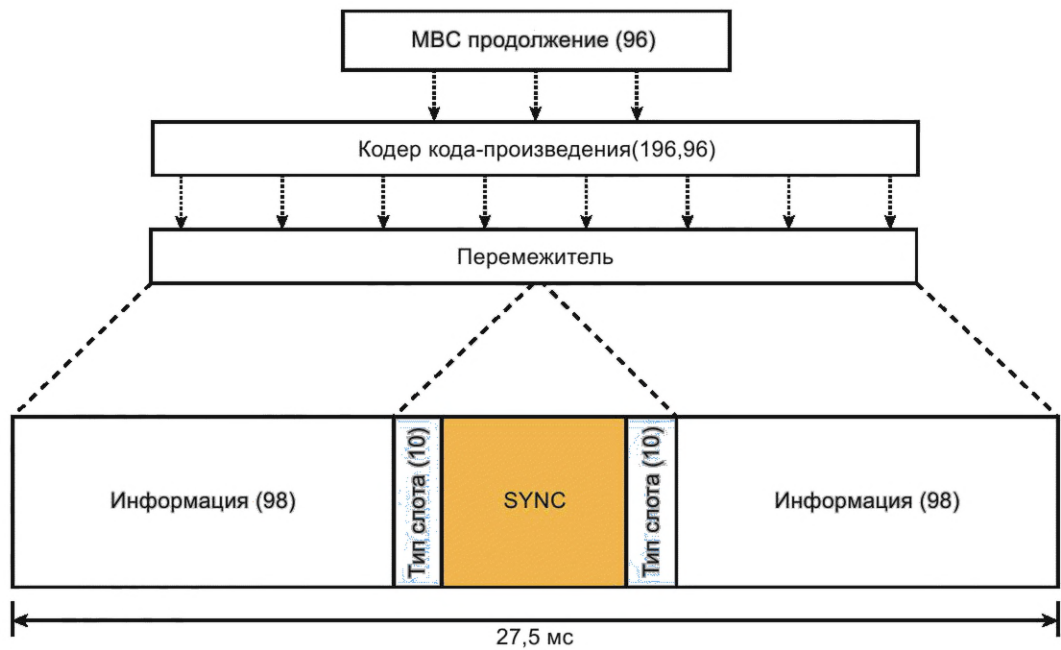
Рисунок 75 — Структура промежуточного блока МВС
