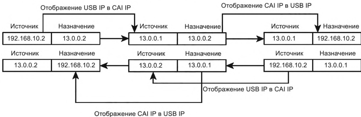
Рисунок А.9 — Цикл NAT-преобразований при двусторонней передаче пакетов внутри IPv4-радиосети
