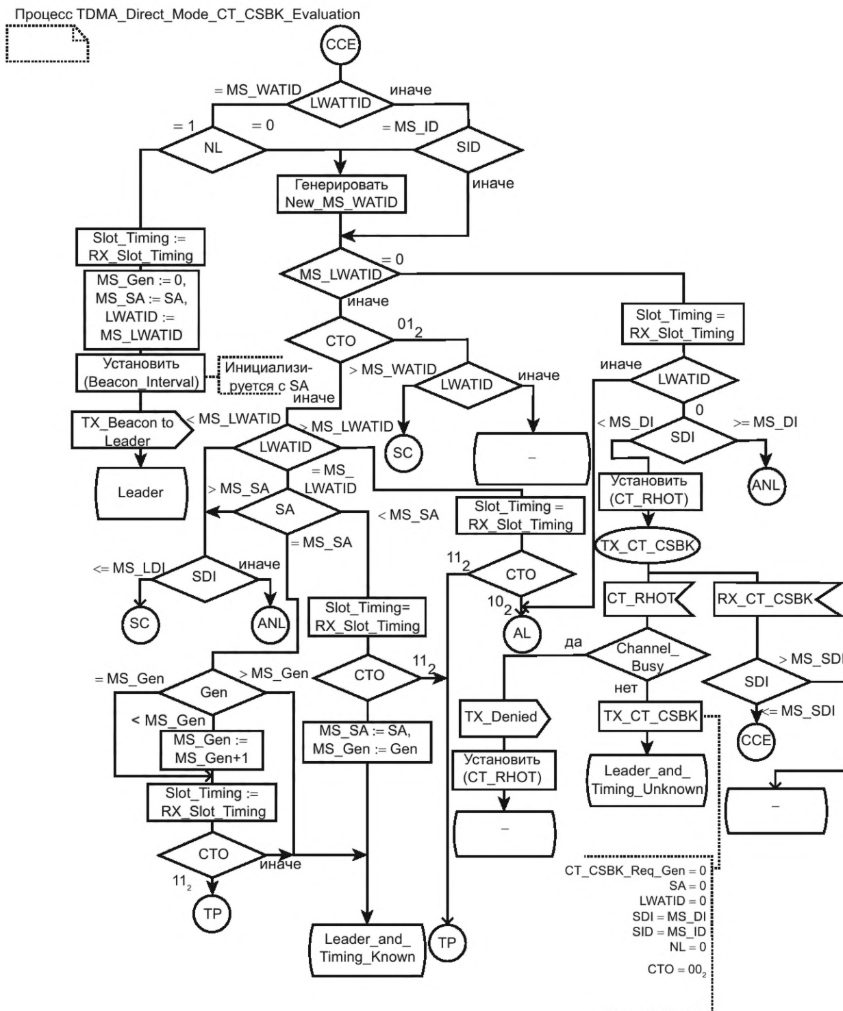
Рисунок 84 — SDL для оценки СТ_CSBK
