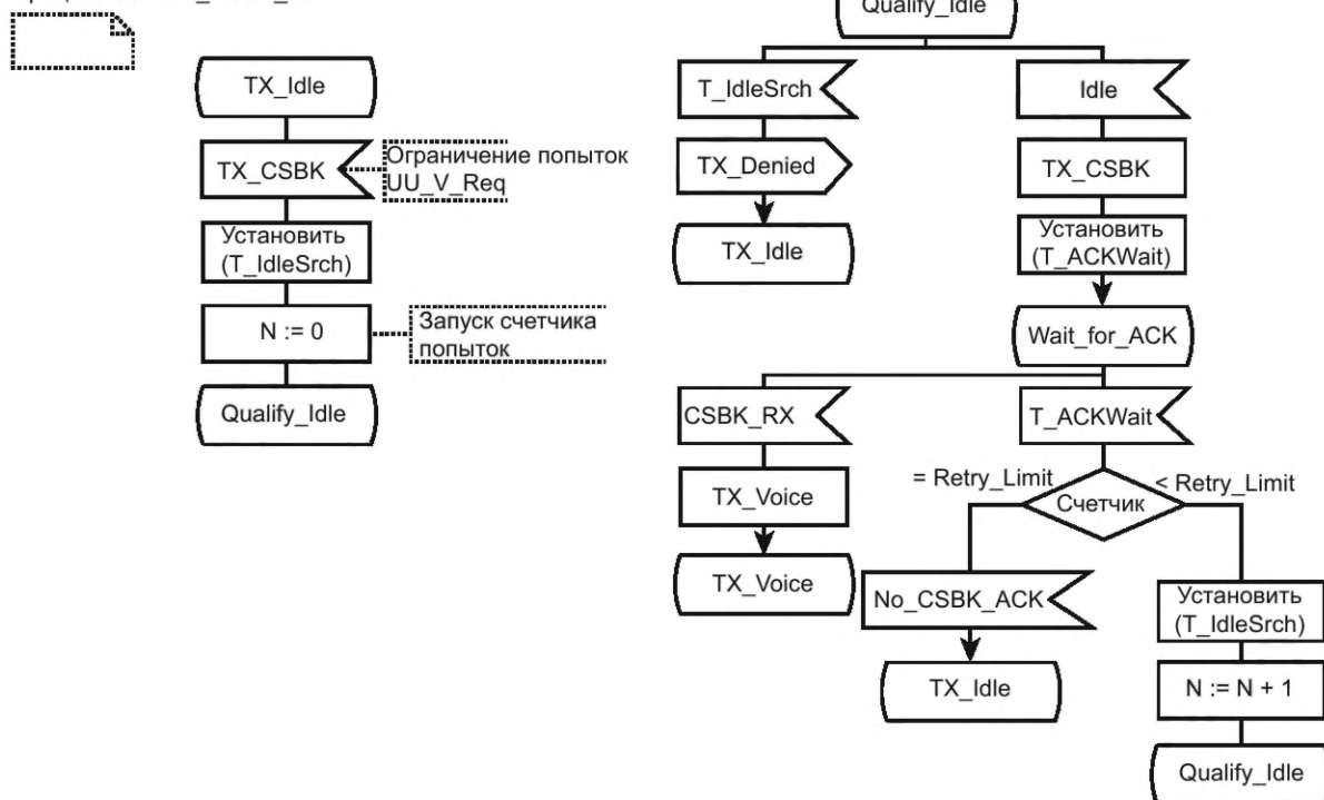
Процесс OACSU_SCBK_TX
