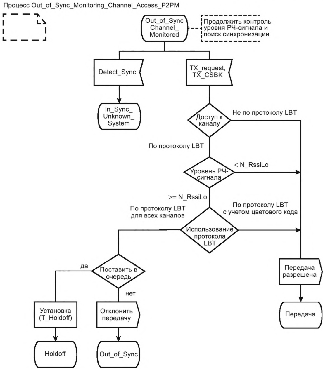
Рисунок 34 — SDL-диаграмма Out_of_Sync_Channel_Monitored
