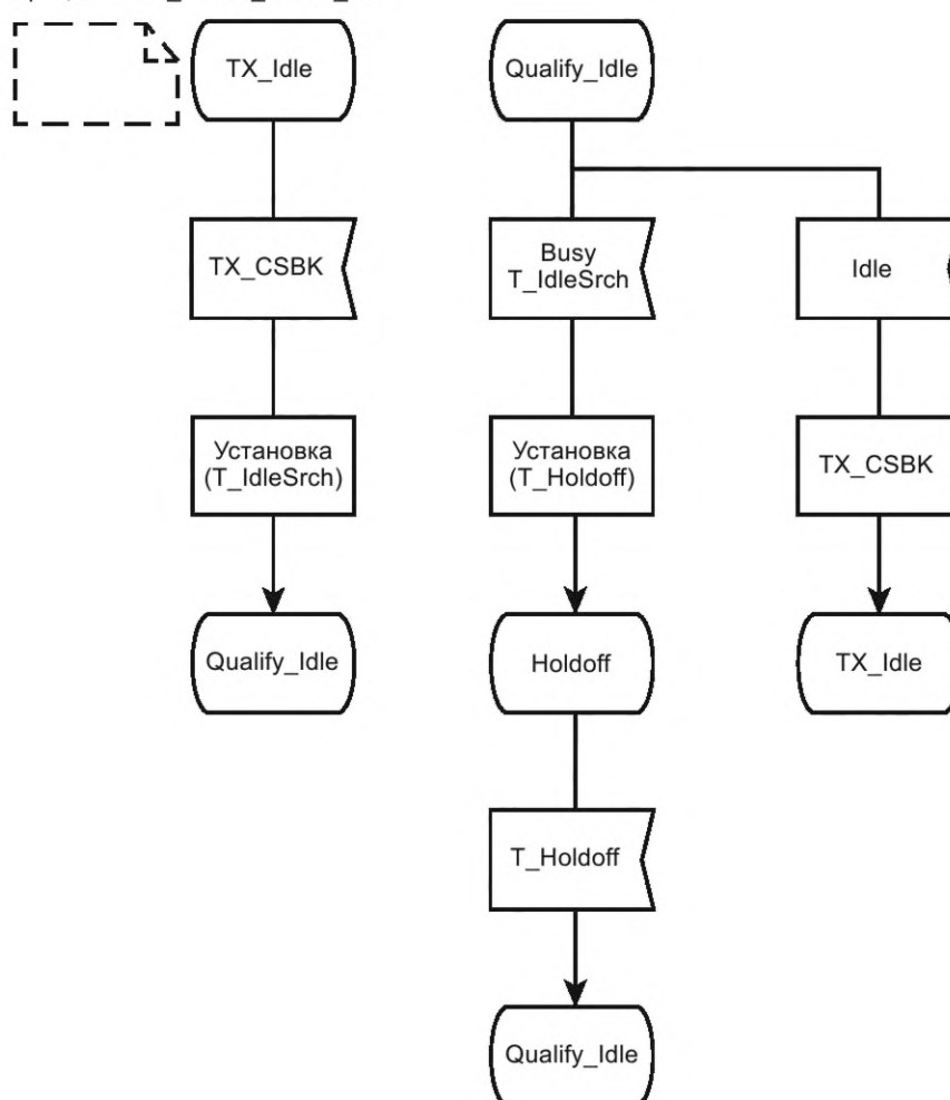
Процесс FNS_NACK_CSBSK_TX
