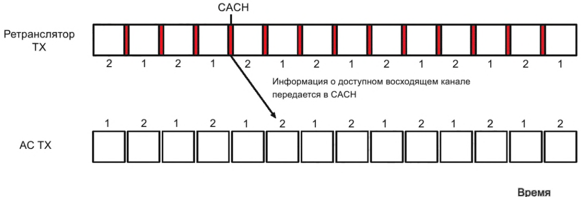
Рисунок 8 — Передача указателя о доступном восходящем канале
