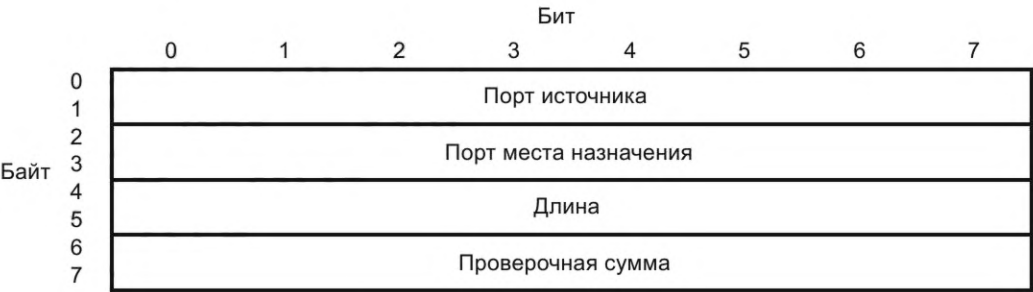
Рисунок 50 — Заголовок UDP
