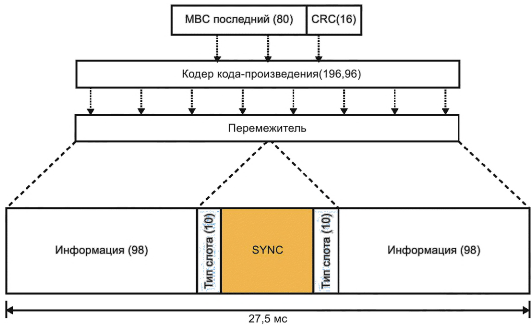
Рисунок 76 — Структура последнего блока МВС
