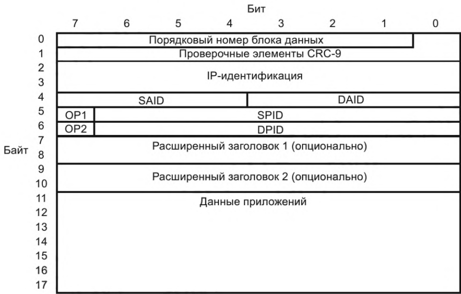
Рисунок 52 — Структура первого блока неподтверждаемых данных с FEC, со скоростью кодирования 1/2 и со сжатием заголовка UDP/IPv4
