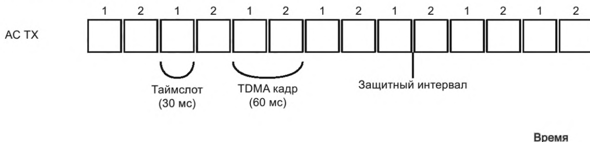
Рисунок 19 — Обобщенная временная диаграмма TDMA
