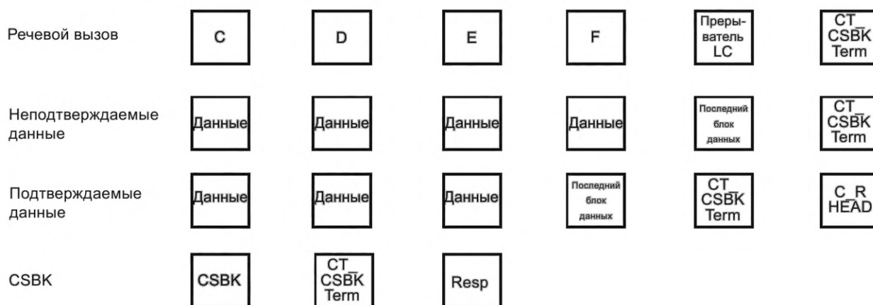
Рисунок 77 — Прерывание с использованием CT_CSBK_Term
