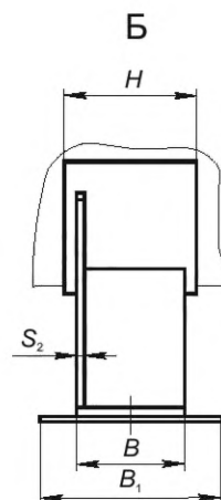
Рисунок 1 — Конструкция подвижной опоры типа 1
