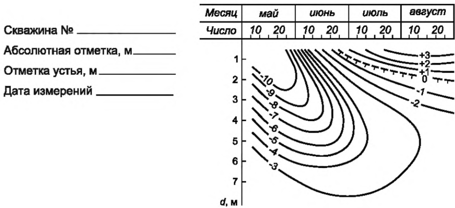
Рисунок Г.2 — Пример графика термоизоплет (термохроноизоплет) для скважины глубиной d по данным стационарных (длительных) температурных наблюдений
