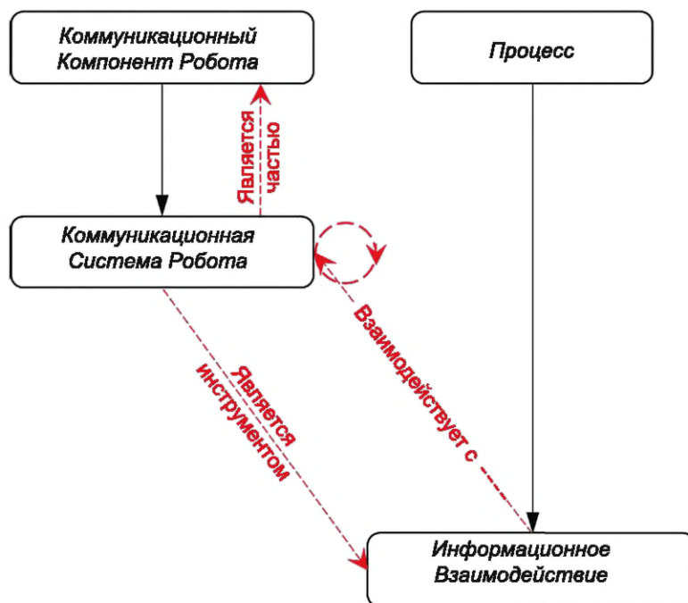
Рисунок 5 — Таксономия понятия Информационное взаимодействие Роботов
