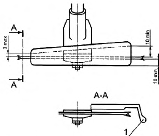
Рисунок 2 — Осевой зазор
