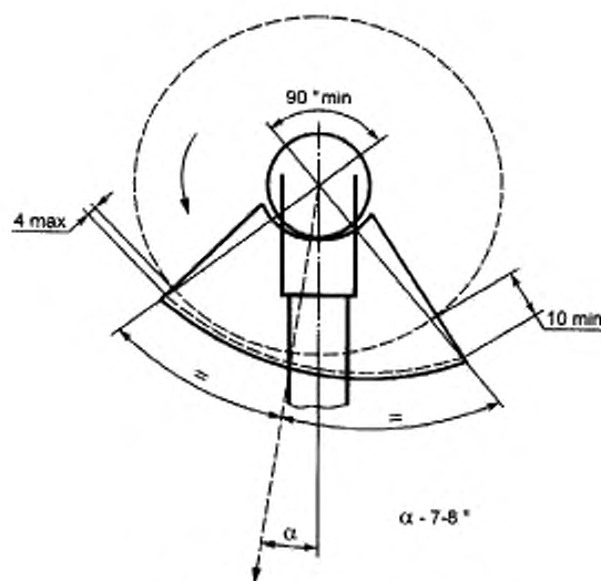
Рисунок 1 — Радиальные зазоры
