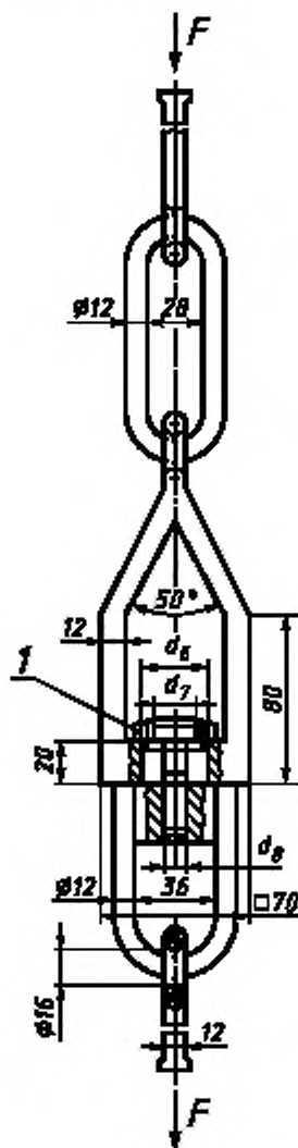
Рисунок 2 — Образец приспособления для испытания на растяжение Т
