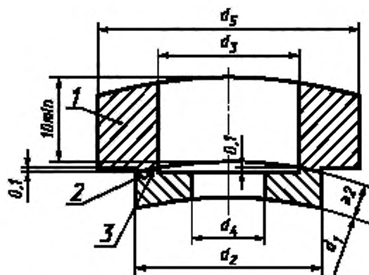
1 — основа; 2 — подшипниковый металл; 3 — поверхность соединения — испытываемая поверхность
