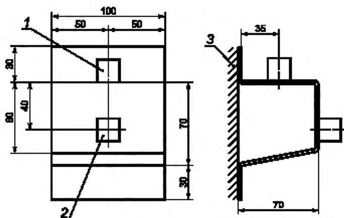
Рисунок Г.4 — Крепление для внутренних выключателей
