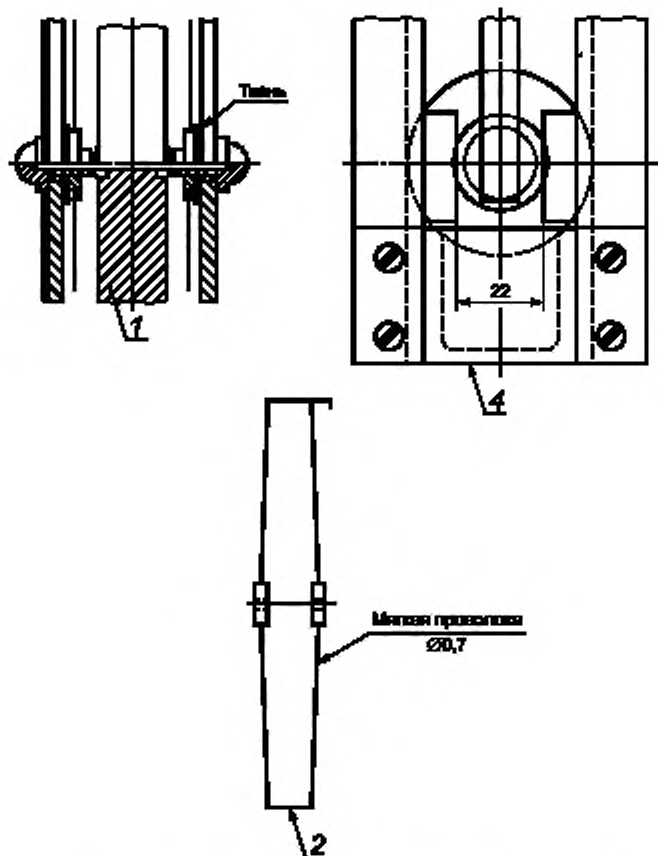
1 — ось; 2 — маркер; 4 — ячейка для спускового устройства
