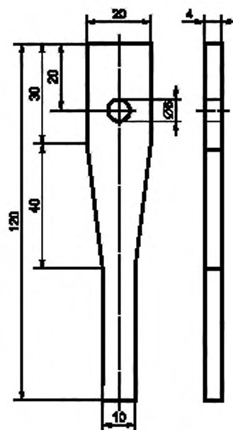
Рисунок Б.3 — Стальная пружина маятника
