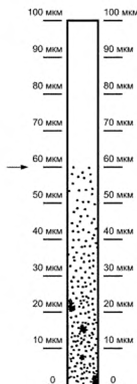
Рисунок 3 — Вид прибора с испытанным образцом
