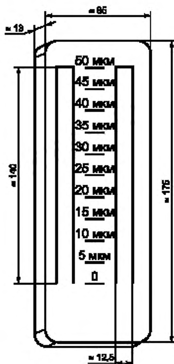
Рисунок 1 — Типовой прибор (грядометр)
