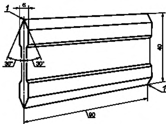
1 — лезвие скребка R 0,25
