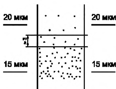
Рисунок 4 — Графическое изображение оценки результатов (частицы); результат — 18 мкм
