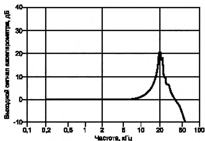
Рисунок 9 — Частичная частотная характеристика акселерометра на магните
