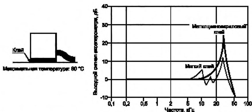
Рисунок 6 — Типичная частотная характеристика акселерометра при клеевом соединении
