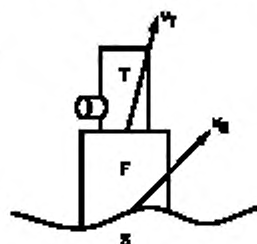
Рисунок 1— Схематическое изображение установки акселерометра
