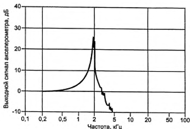
Рисунок 8 — Типичная частотная характеристика акселерометра с щупом
