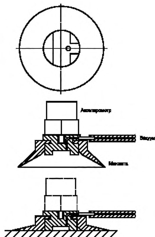
Рисунок 11 — Вакуумное крепление
