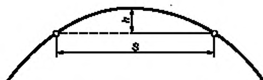
Рисунок 2 — Схема определения радиуса горизонтальной кривой
