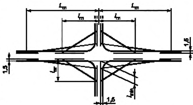
Рисунок 3 — Схема определения боковой видимости
