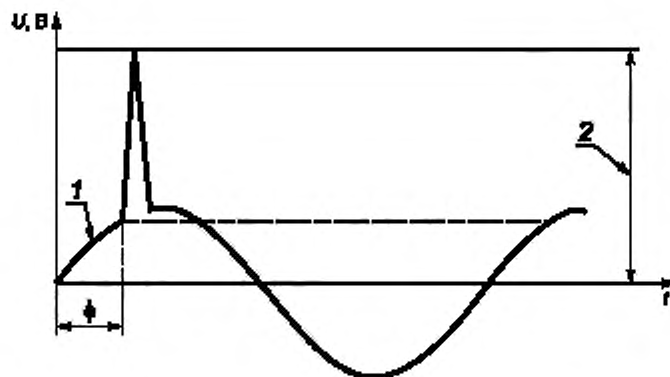
1 — мгновенное напряжение; 2 — пиковое напряжение
