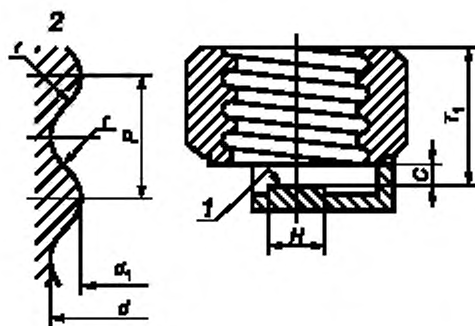
1 — поверхность X; 2 — деталь резьбы (правая резьба)
