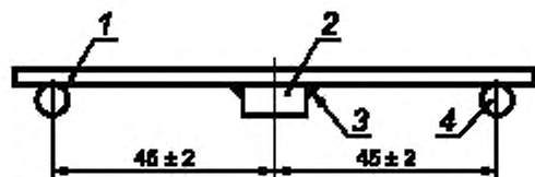
Рисунок 4 — Испытательное основание плавкого предохранителя
