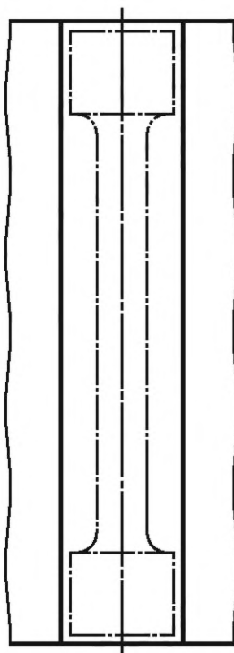
Рисунок 1 — Пример расположения образцов для испытаний. Продольный плоский разрез
