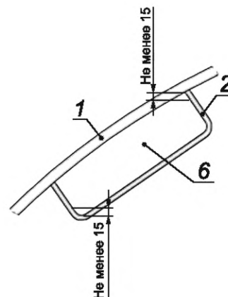
г) Вид продольного желоба в сечении электродегидратора
