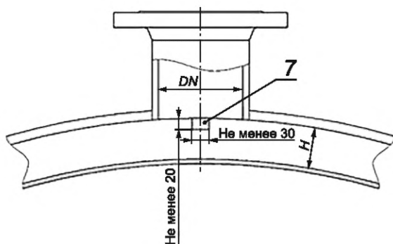
в) Вид штуцера вывода обезвоженного продукта в сечении электродегидратора
