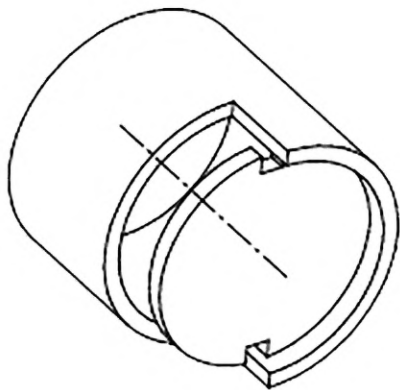
в) Торцевая заглушка, вид с торца в сечении А
