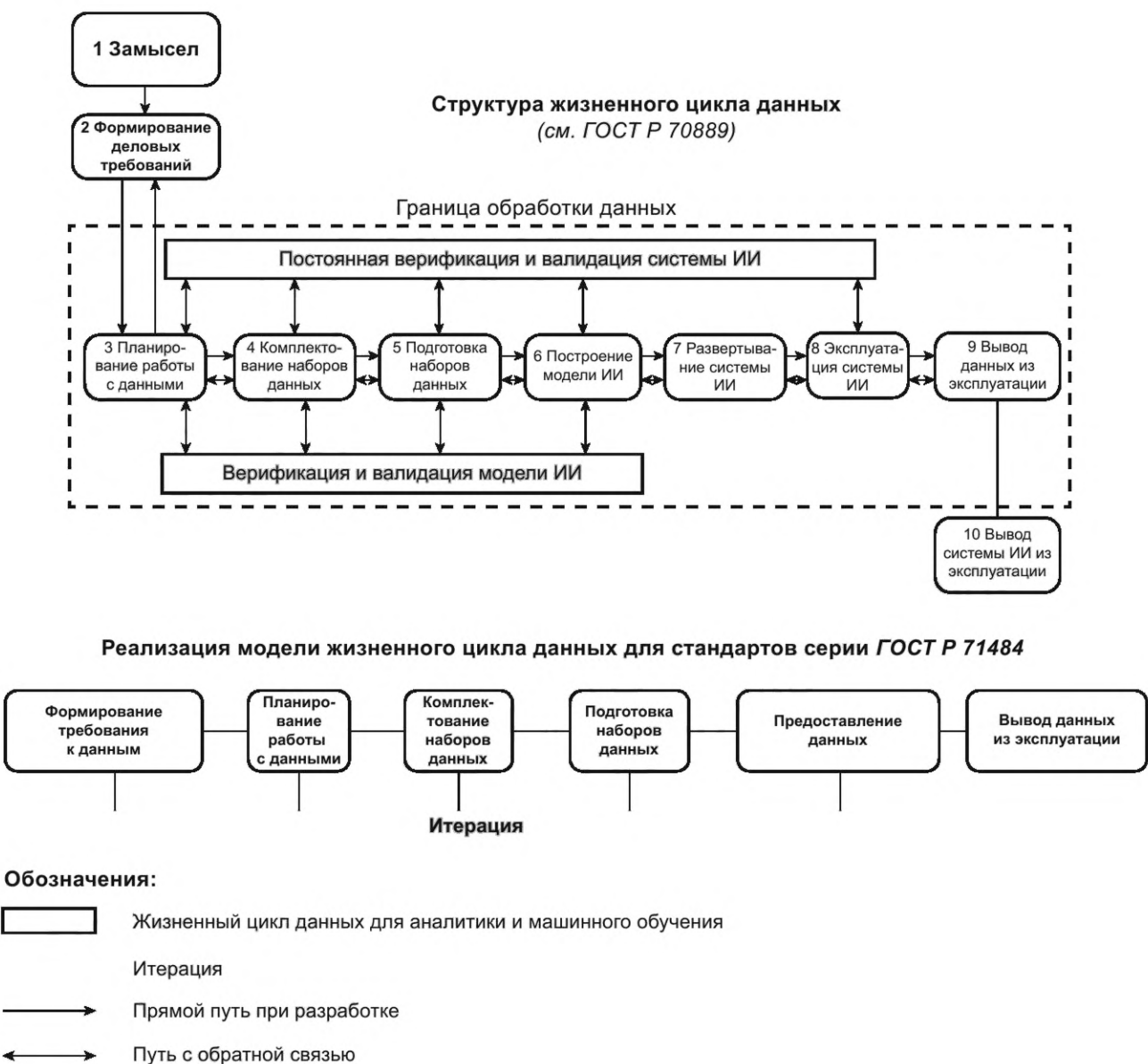
Рисунок 3 — Модель жизненного цикла данных для аналитики и машинного обучения
