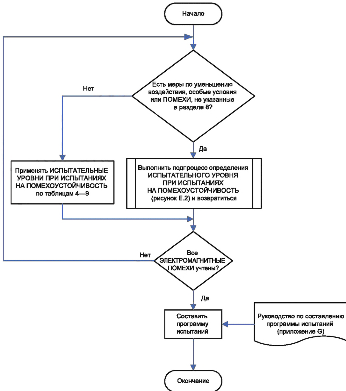
Рисунок E.1 — Процесс разработки программы испытаний, если указаны ОСОБЫЕ ОБСТАНОВКИ
