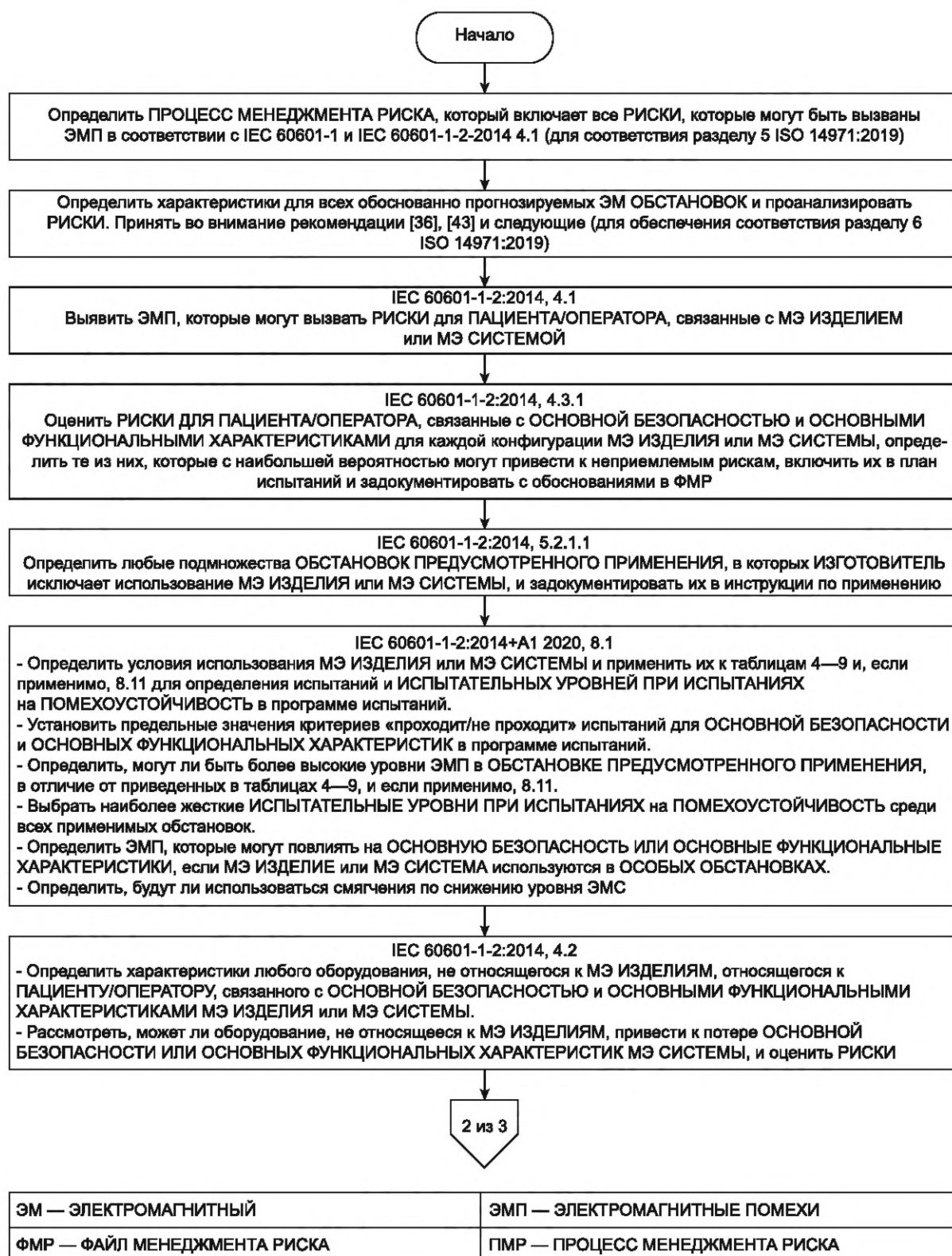
Рисунок F.1 — Процесс менеджмента риска в IEC 60601-1-2 (1 из 3)
