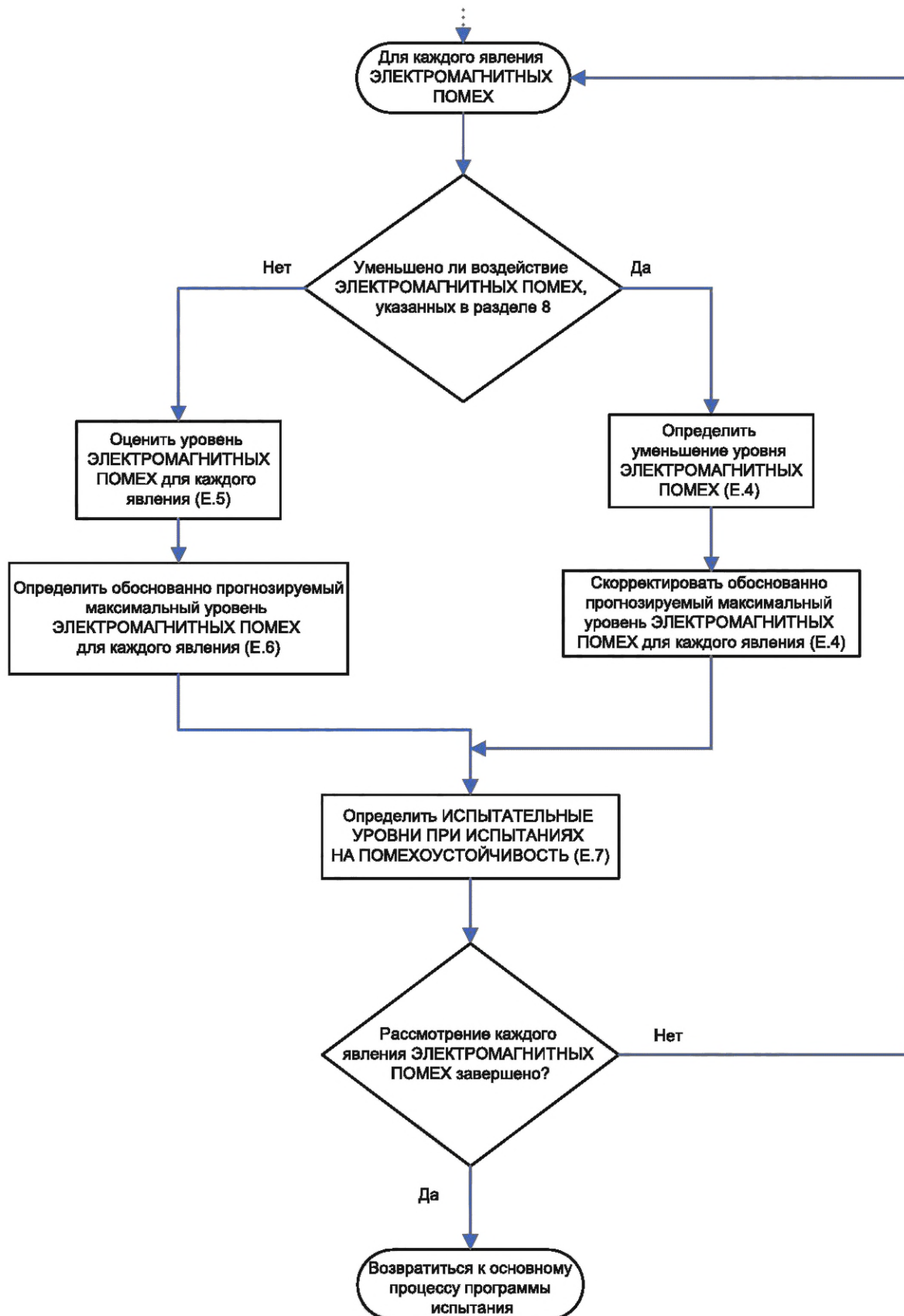
Рисунок Е.2 — Подпроцесс определения ИСПЫТАТЕЛЬНЫХ УРОВНЕЙ ПРИ ИСПЫТАНИЯХ НА ПОМЕХОУСТОЙЧИВОСТЬ для ОСОБЫХ ОБСТАНОВОК
