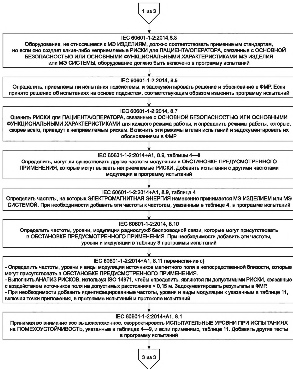
Рисунок F.2 — Процесс менеджмента риска в IEC 60601-1-2 (2 из 3)
