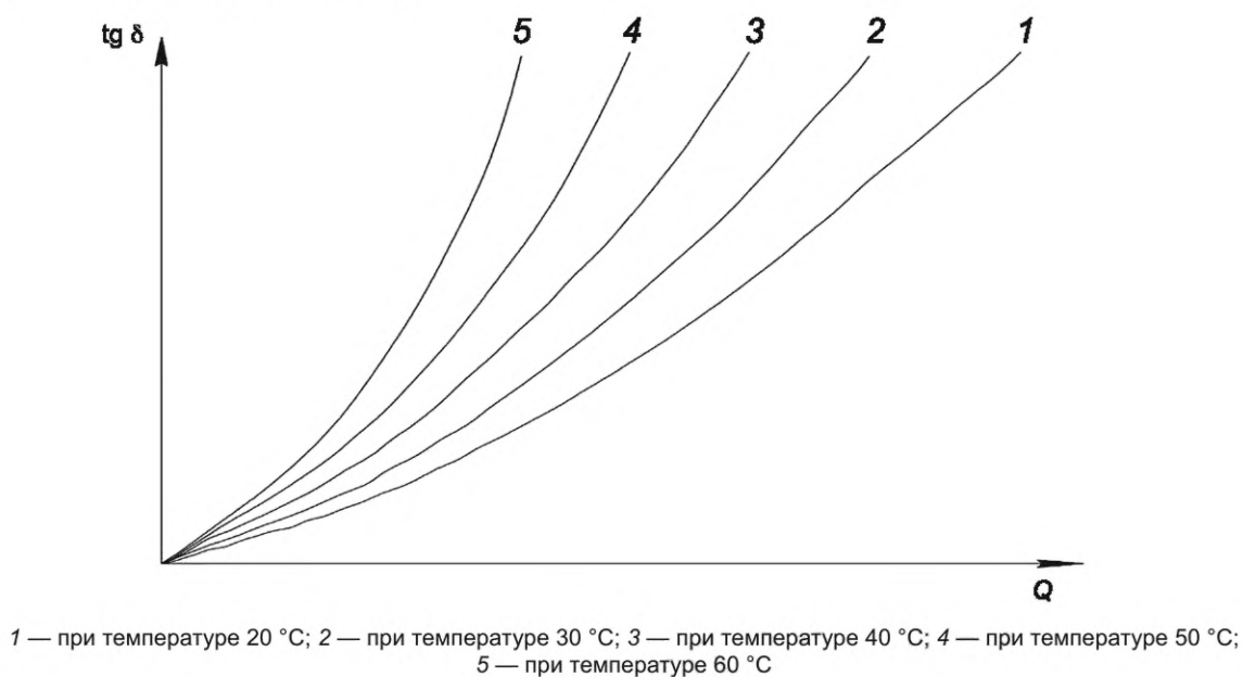
Рисунок 3 — Зависимость тангенса угла диэлектрических потерь индикатора \text{tg } \delta от количества поглощенной им влаги при разных температурах
