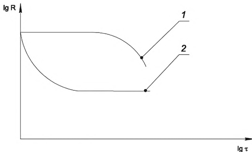
Рисунок 5 — Зависимость сопротивления на поверхности испытуемого образца от времени при оценке сорбционных свойств материала
