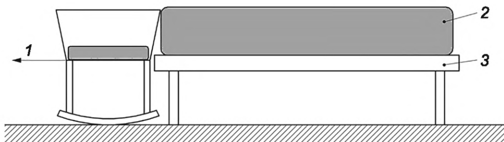
1 — направление приложения усилия; 2 — испытательная платформа — матрас для испытаний; 3 — испытательная платформа — основание матраца
