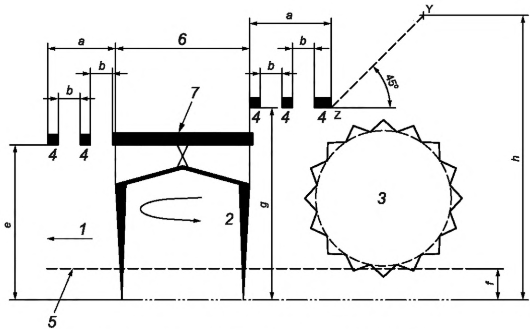
с) Заднее защитное устройство (см. 4.3.2 b), первое перечисление)
