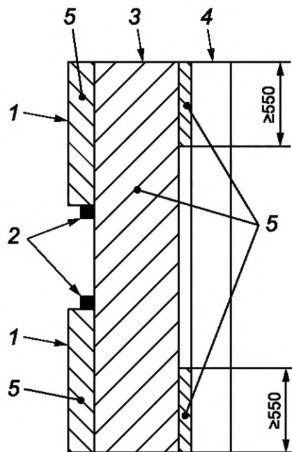
1 — передний барьер; 2 — нижние точки навески; 3 — рабочий орган с механическим приводом (траектория движения рабочего органа); 4 — устройство, препятствующее доступу; 5 — область, которая должна быть проверена в соответствии с разделом 5
