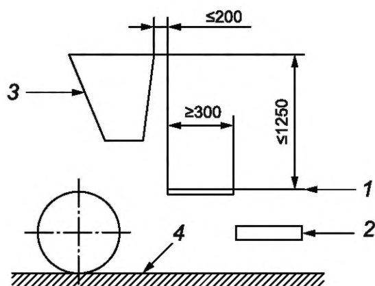
Рисунок 4 — Размеры средств доступа к зоне загрузки при наличии платформы
