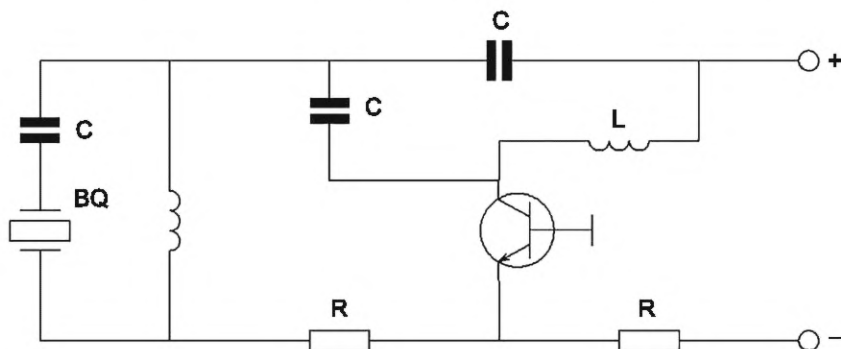
Рисунок В.4 — Генератор по схеме Колпитца до 300 МГц (резонатор в цепи обратной связи)
