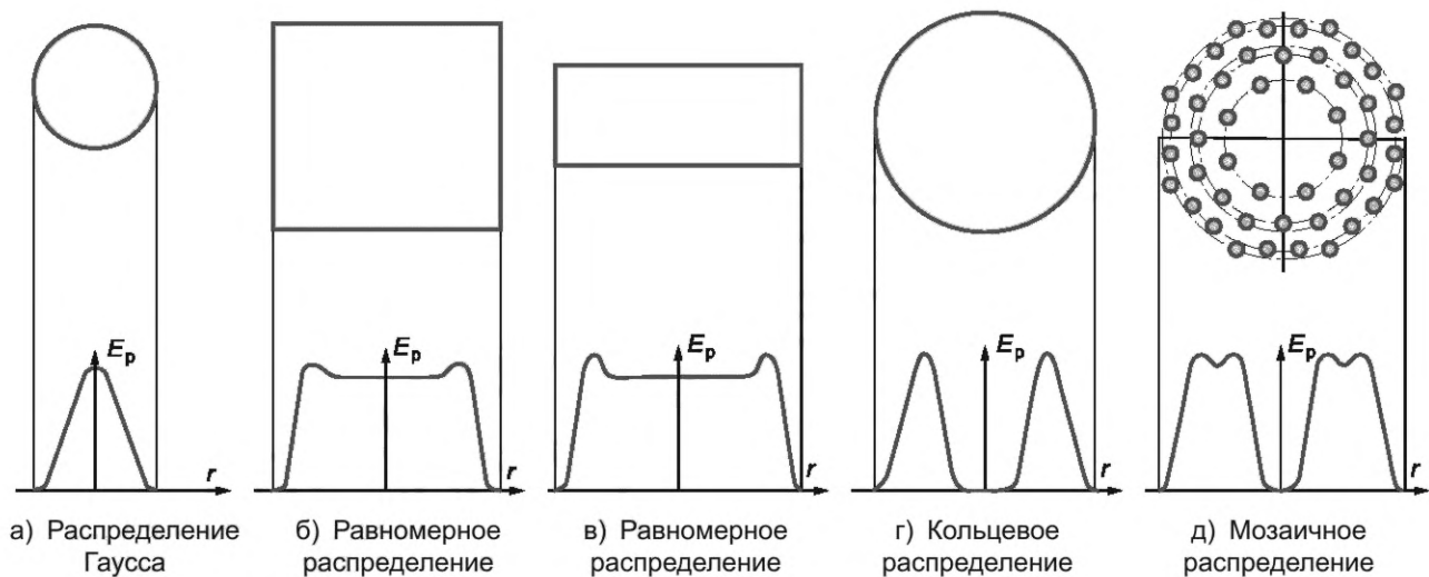
Рисунок 4 — Распределение плотности мощности лазерного излучения E_p
