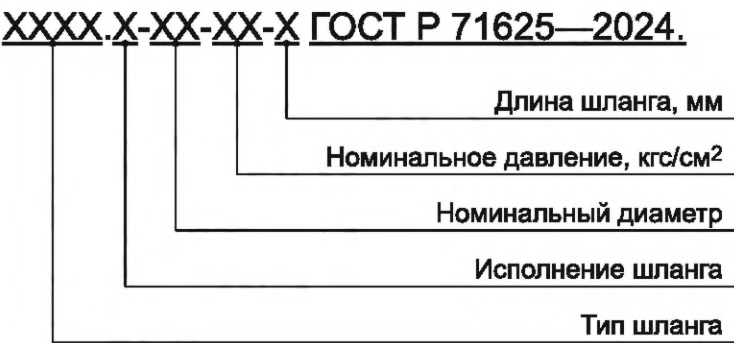
Рисунок 15 — Схема условных обозначений шлангов
