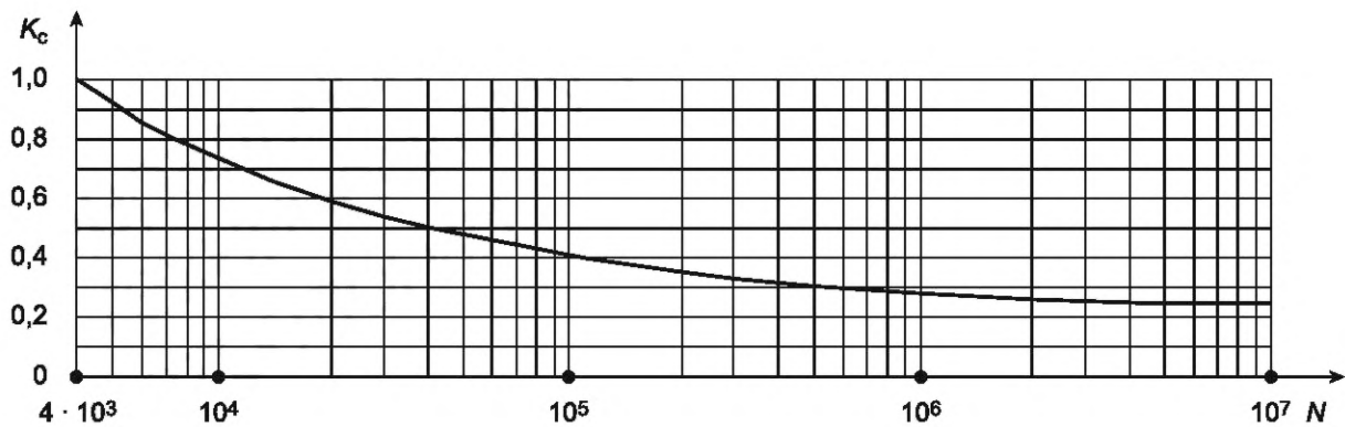
N — наработка, циклы; K c — коэффициент, учитывающий изменение амплитуды перемещения
