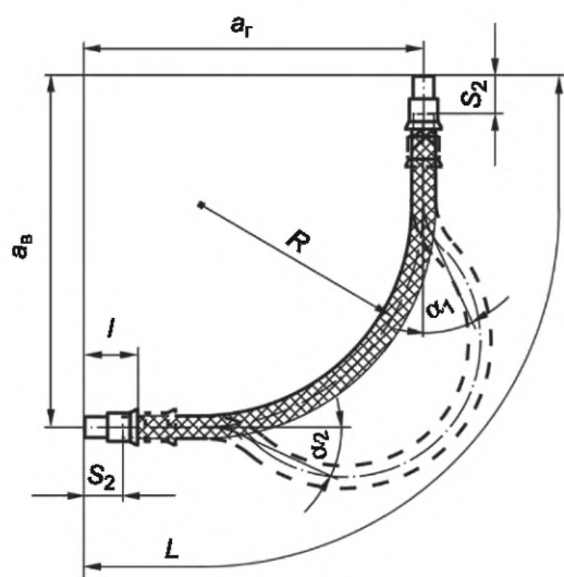
Рисунок Д.10 — Схема монтажа для компенсации перемещения двух концов шланга в направлении вдоль его оси при малой частоте перемещения (без вибрации)
