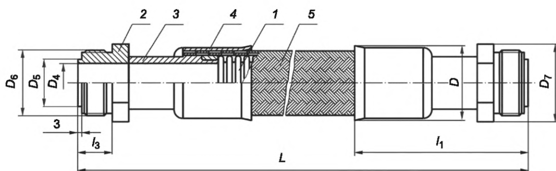
1 — гофрированная труба; 2 — штуцер; 3 — наконечник; 4 — втулка; 5 — оплетка
