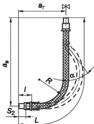
Рисунок Д.8 — Схема монтажа для компенсации перемещения конца шланга в направлении, вдоль его оси при малой частоте перемещения (без вибрации)
