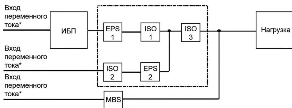
Рисунок С.2 — Внутренний байпасный переключатель для технического обслуживания
