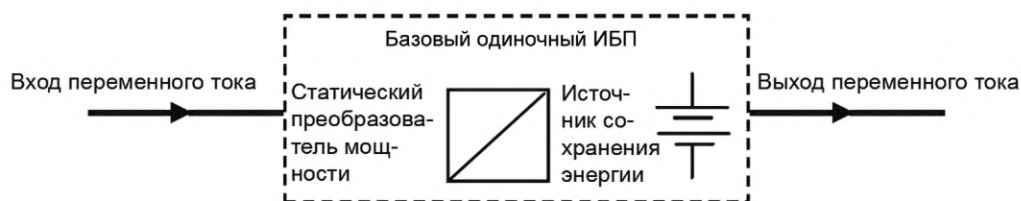
Рисунок А.1 — Одиночный ИБП — базовый
