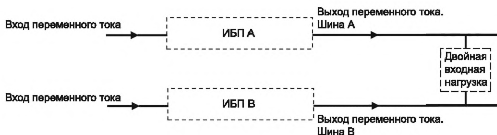
Рисунок А.6 — ИБП с двумя шинами
