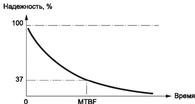
Рисунок К.1 — График зависимости надежности, %, от времени
