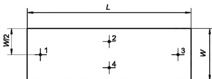
Рисунок 3 — Точки измерения толщины предметного стекла
