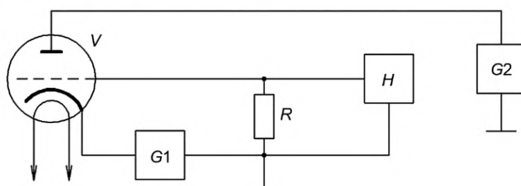
G1, G2 — источники питания индикационного устройства; H — индикационное устройство; R — измерительный резистор; V — испытательная лампа
