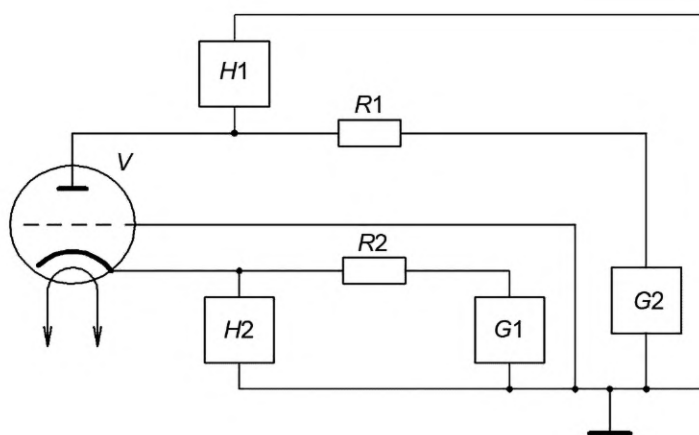
G1, G2 — источники питания индикационного устройства; H1, H2 — индикационные устройства; R1, R2 — измерительные резисторы; V — испытательная лампа
