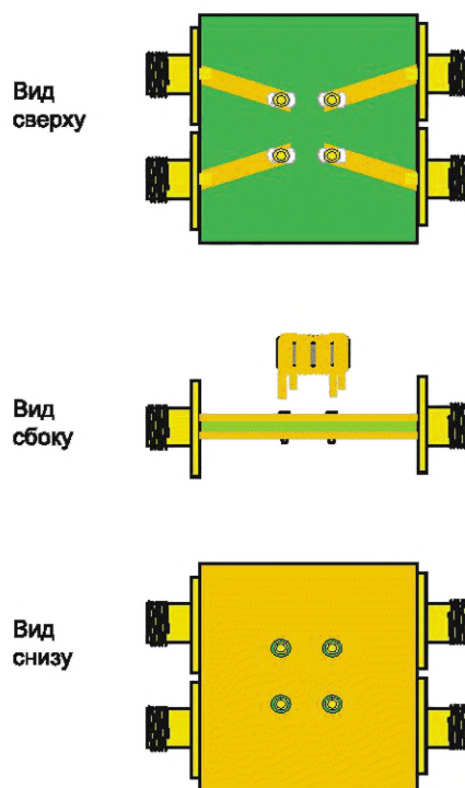
Рисунок G.10 — Испытательное устройство для S-параметров четырех портов оборудования с выводами
