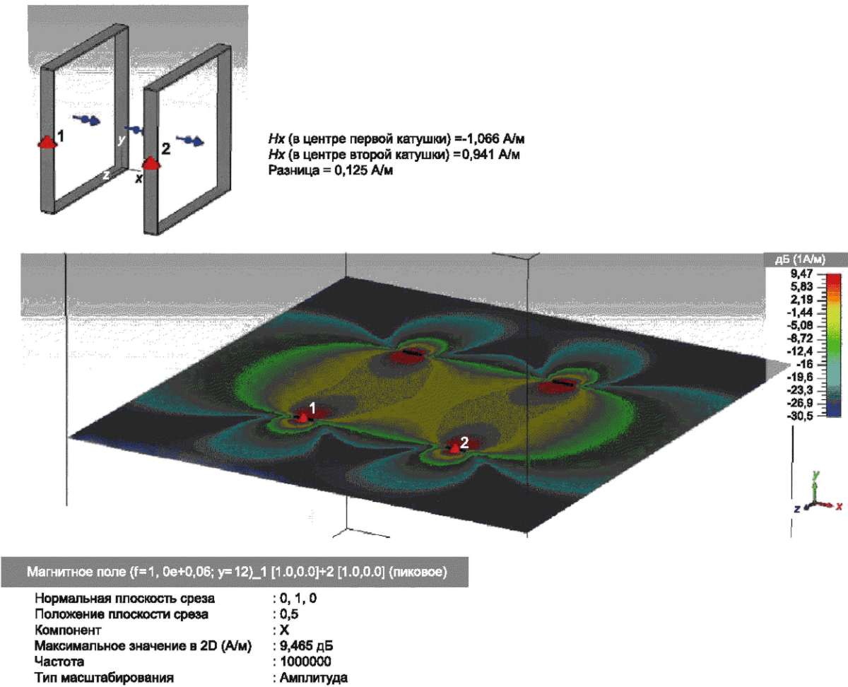
Рисунок G.12 — Установка Гельмгольца: магнитное поле H_x и двумерный график для двух индукционных катушек размером 1 × 1 м, расстояние между которыми 0,8 м
