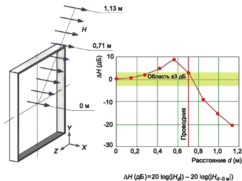
Рисунок G.5 — Значение магнитного поля H_x , дБ, вдоль диагонали для индукционной катушки размером 1 \times 1 м
