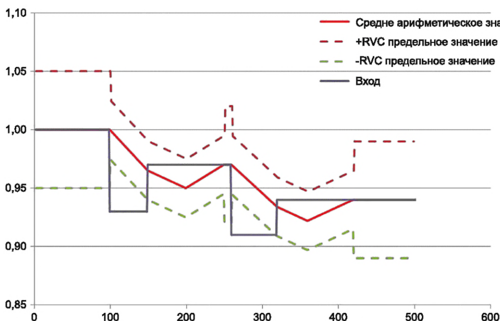
Рисунок 33 — Форма сигнала вместе с RVC-предельными значениями и средним арифметическим значением по A13.5.2
