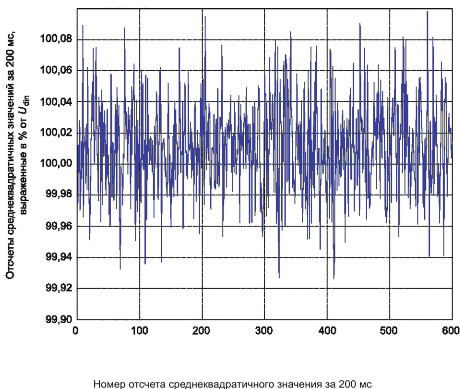
Рисунок G.1 — Моделирование сигнала в условиях шумов
