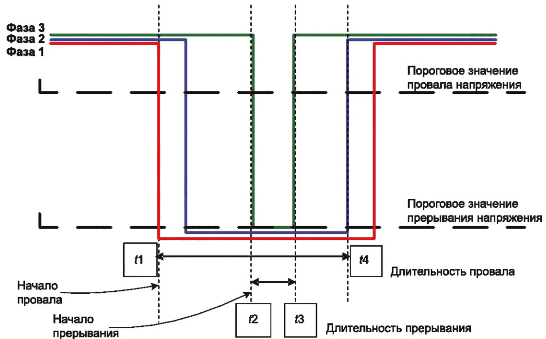
Рисунок 11 — Первая детализация формы сигнала при испытании на провалы/прерывания напряжения в многофазных системах
