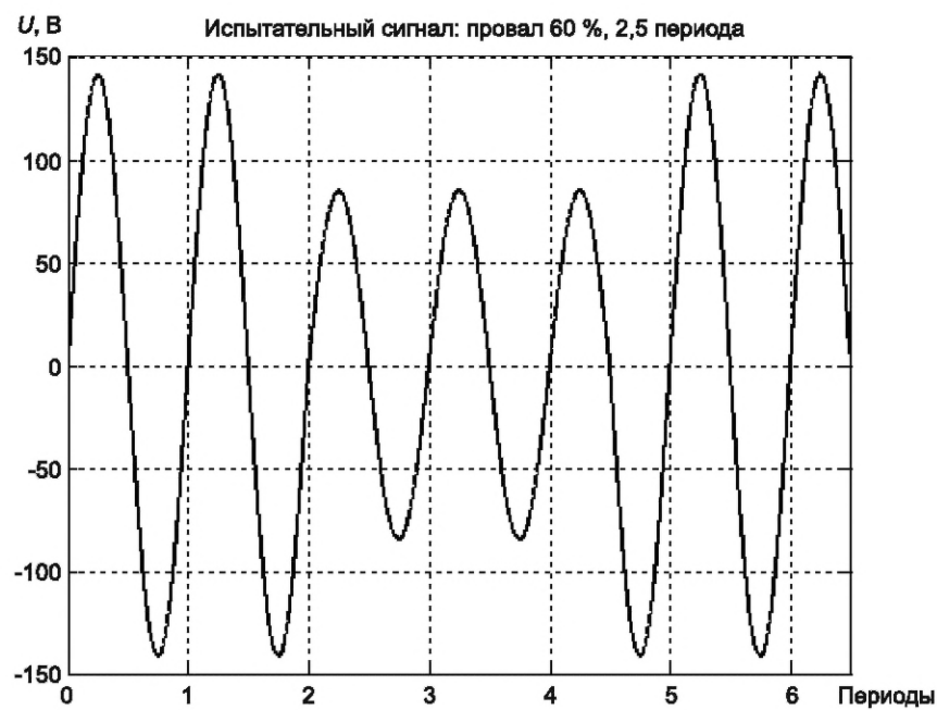
Рисунок 34 — Первая детализация формы сигнала при испытании на провалы напряжения в соответствии с испытанием S4.1.2
