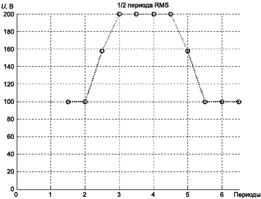
Рисунок 37 — Вторая детализация формы сигнала при испытании на перенапряжения в соответствии с испытанием S4.1.2
