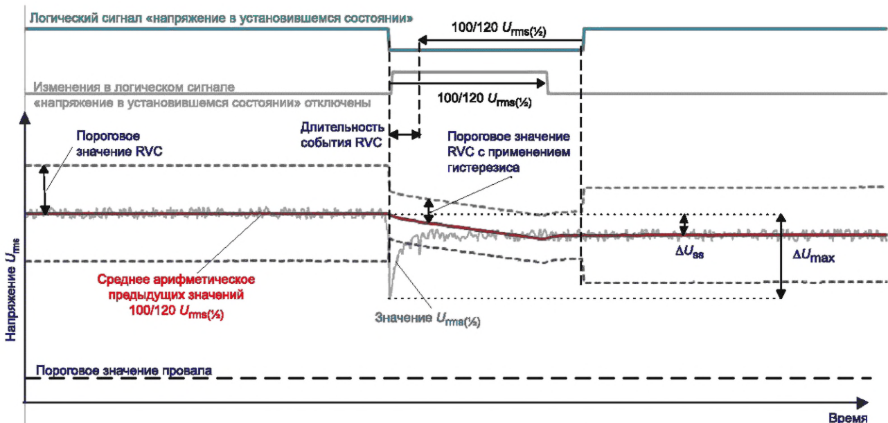
Рисунок 18 — Пример события RVC
