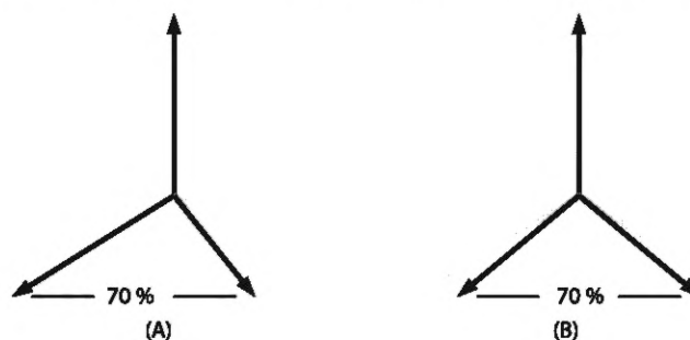
Рисунок D.1 — Испытание «фаза—нейтраль» в трехфазных системах
