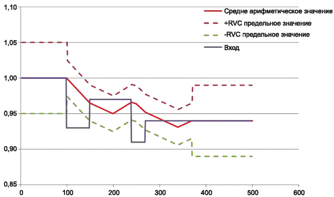
Рисунок 31 — Форма сигнала вместе с RVC-предельными значениями и средним арифметическим значением по A13.5.1
