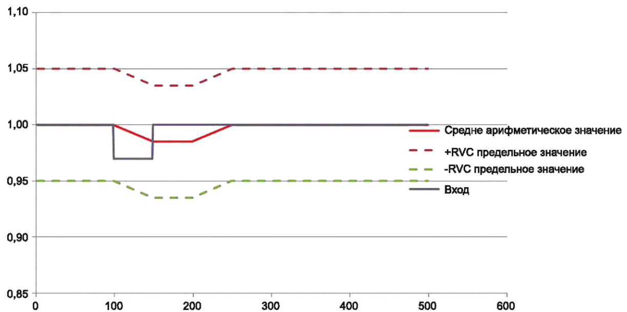
Рисунок 22 — Форма сигнала вместе с RVC предельными значениями и средним арифметическим значением по A13.1.2
