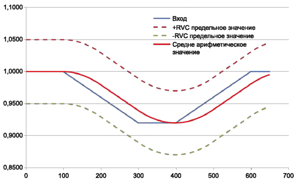
Рисунок 19 — Форма сигнала по A13.1.1
