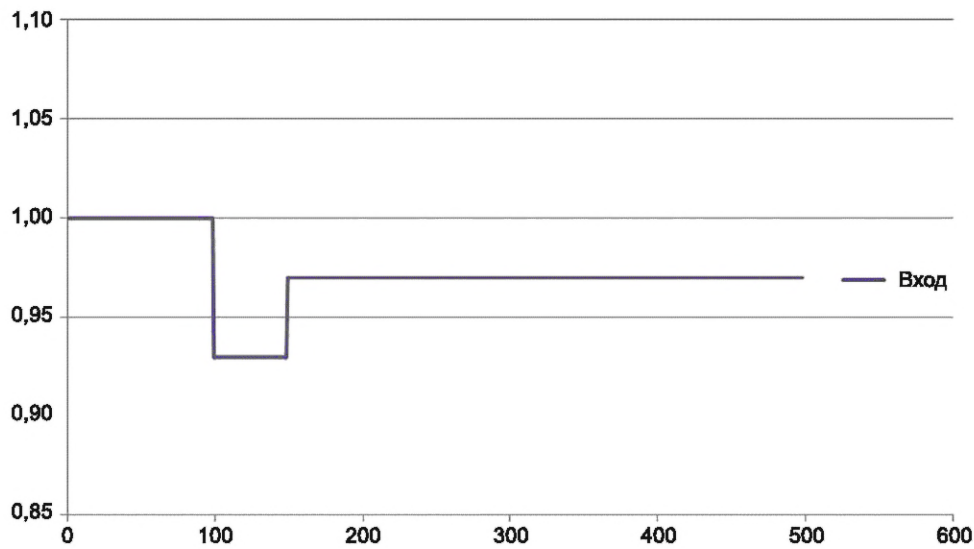
Рисунок 27 — Форма сигнала по A13.3.1
