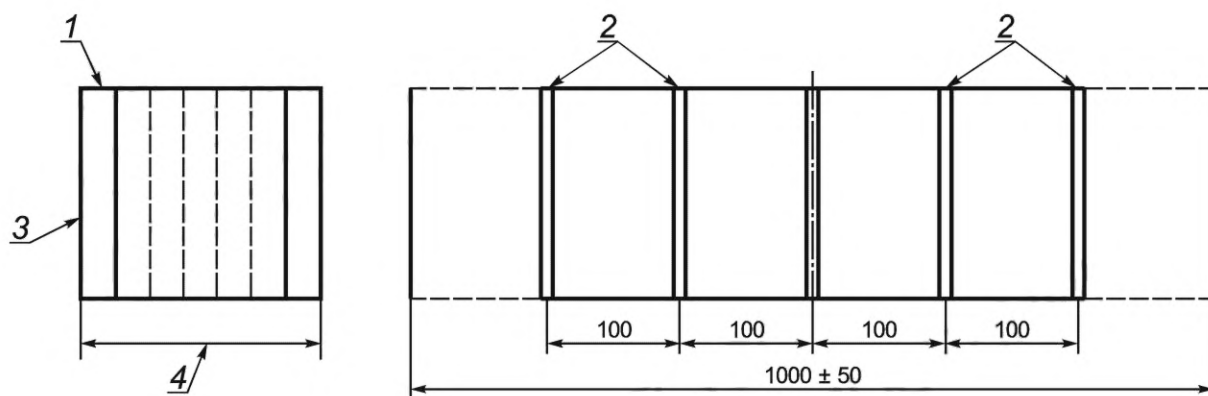
1 — меньшая ось кабеля; 2 — проволочный бандаж; 3 — большая ось кабеля; 4 — n -е количество испытуемых отрезков
