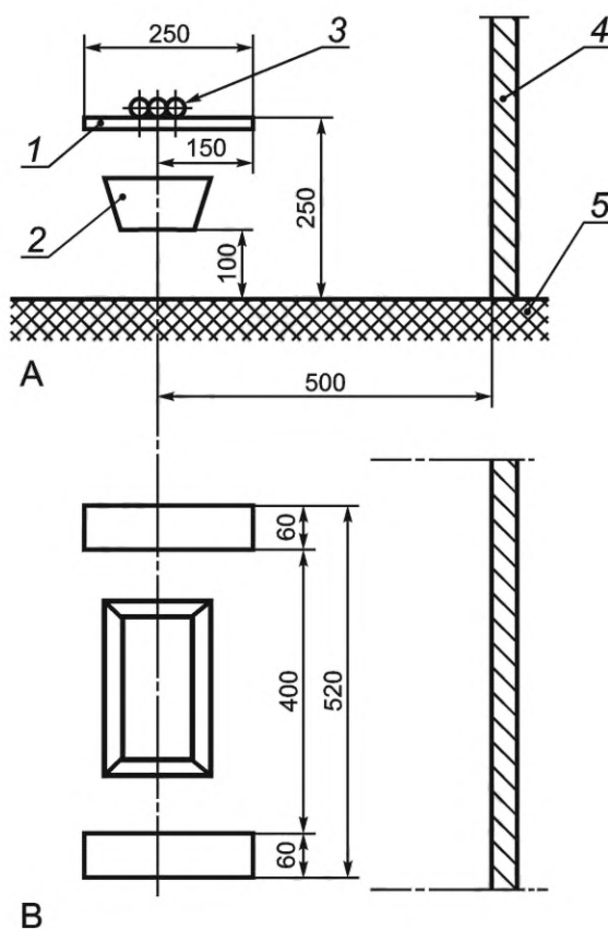
А — вид сбоку; В — вид сверху; 1 — опора; 2 — металлический поддон; 3 — испытуемый образец; 4 — задняя стенка; 5 — пол Рисунок 2 — Расположение образцов на опоре
