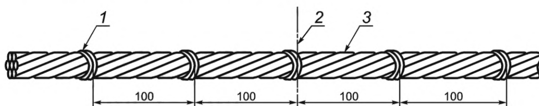
1 — проволоочный бандаж; 2 — центр; 3 — пучок из семи отрезков кабеля
