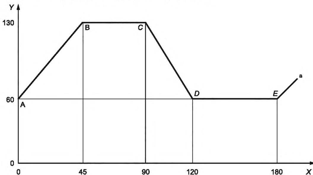
Рисунок 1 — Термоциклы
