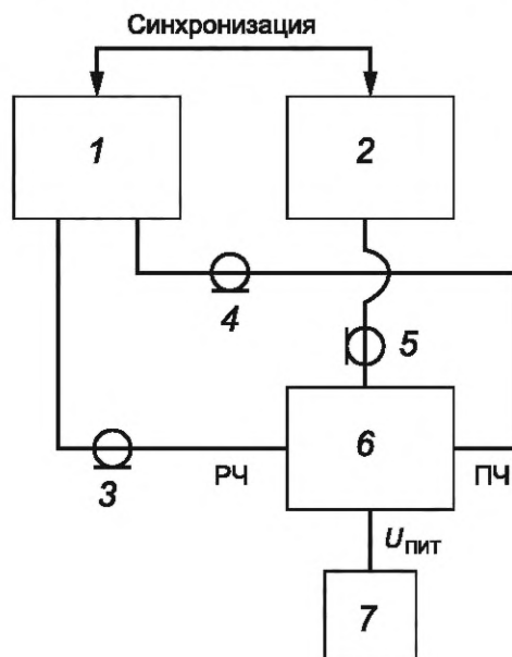
1 — ВАЦ; 2 — ГН; 3, 4, 5 — КС; 6 — ИУ; 7 — ИП
