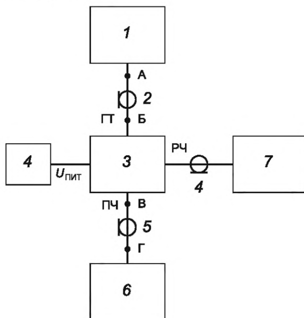
Рисунок 8 — Структурная схема стенда для измерения развязки между каналами гетеродина и промежуточной частоты
