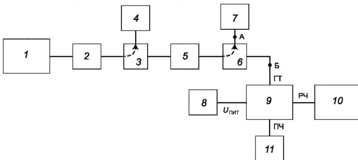
1 — ГН; 2 — изолятор; 3 — направленный ответвитель; 4 — измеритель частоты; 5 — регулируемый аттенюатор; 6 — направленный ответвитель; 7 — измеритель мощности; 8 — ИП; 9 — ИУ; 10 — АС; 11 — согласованная нагрузка
