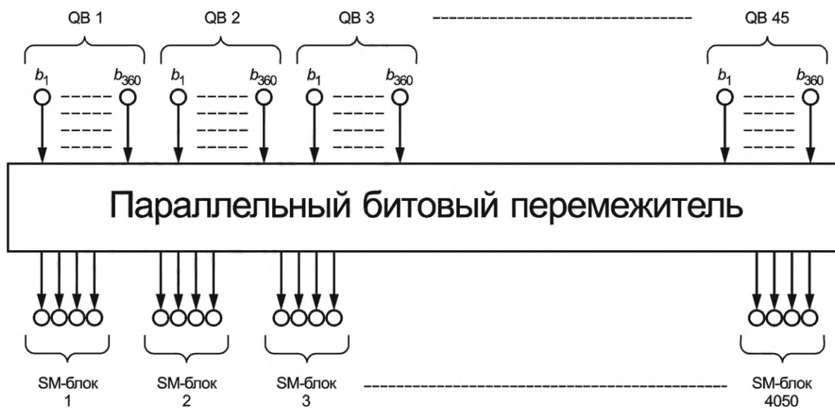
Рисунок 7 — Структурная схема параллельного битового перемежителя для N_{\text{bpsu}} = 8
