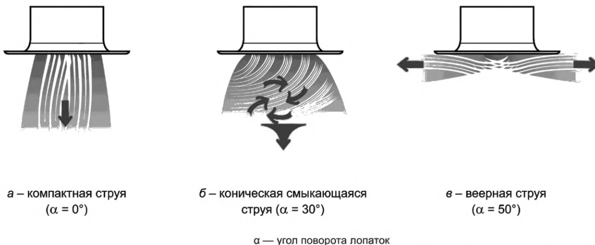
Рисунок 2 — Пример представления видов струй, формируемых диффузором с поворотными лопатками
