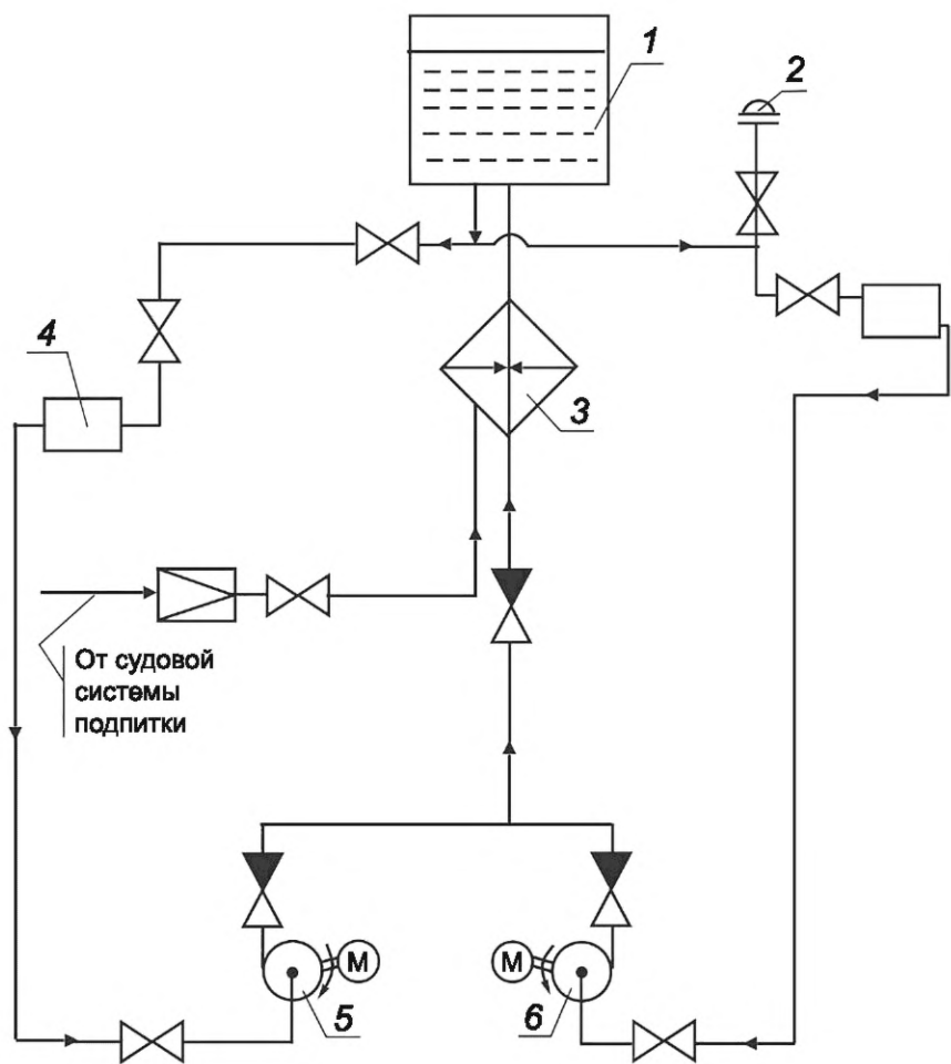
1 — расширительная цистерна; 2 — воздушный клапан; 3 — теплогенератор; 4 — отопительный прибор; 5, 6 — циркуляционный насос
