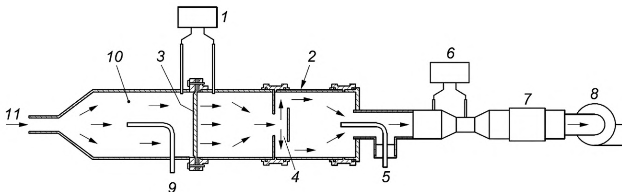
1 — манометр; 2 — испытательный канал; 3 — образец фильтрующего материала; 4 — смесительная секция; 5 — проботоотборная трубка после фильтра; 6 — расходомер; 7 — устройство контроля расхода воздуха; 8 — вентилятор; 9 — проботоотборная трубка до фильтра; 10 — канал до фильтра; 11 — контрольный аэрозоль
