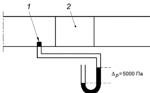
1 — заглушенное отверстие для измерения давления; 2 — секция испытательного устройства
