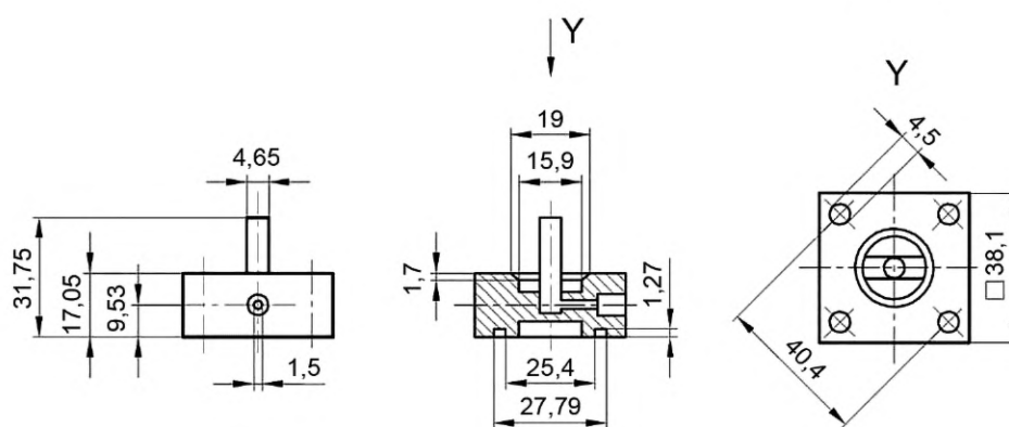
в) Эжектор Вентури
