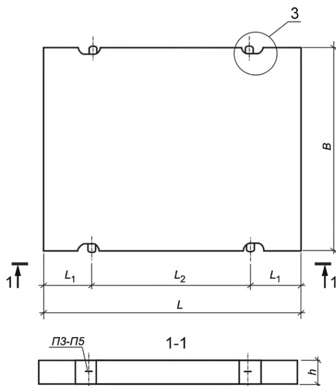
Рисунок А.3 — Плиты ПЗ5.28, ПЗ0.18, П18.18, П18.15
