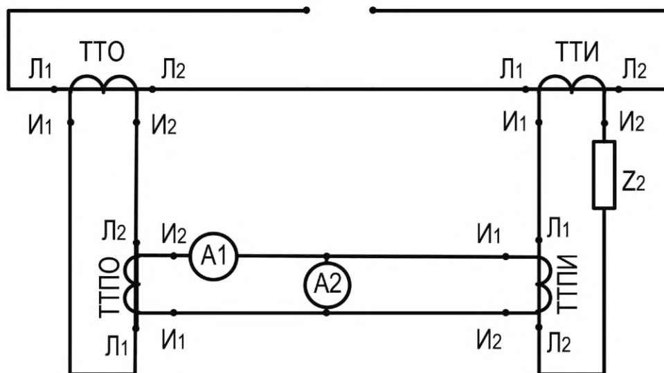
A1 — амперметр для измерения испытательного тока; A2 — амперметр для измерения тока погрешности; Z_2 — вторичная нагрузка в цепи испытуемого ТТ
