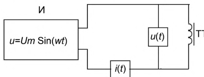
Рисунок В.1 — Схема испытаний от источника синусоидального напряжения
