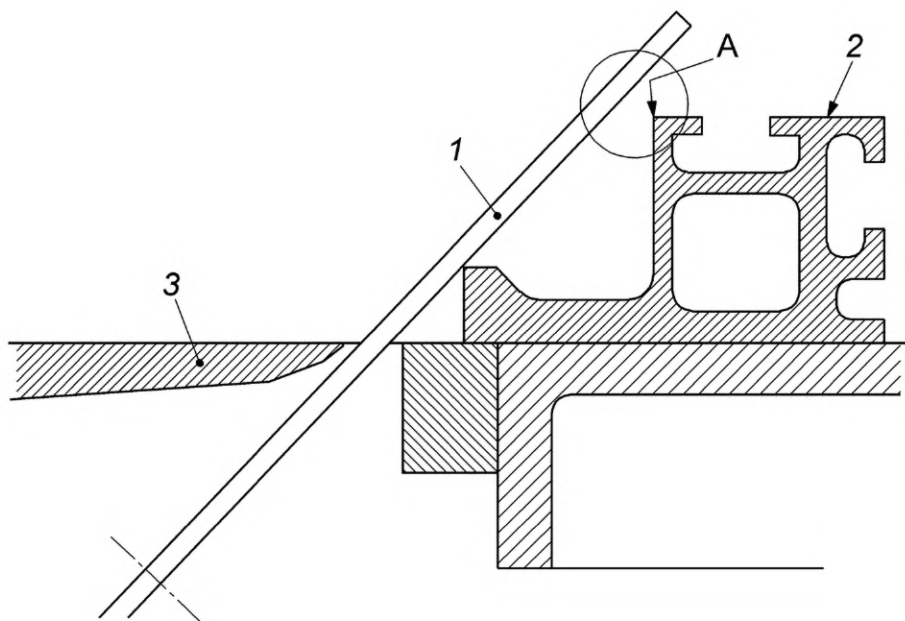
1 — дисковая пила в положении максимального наклона; 2 — направляющая планка в нижнем положении; 3 — стол станка; А — указанная точка касания
