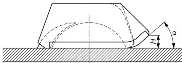
\alpha — угол скоса; H — высота скоса
