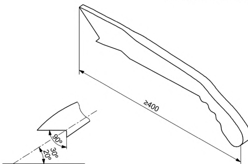
Рисунок 24 — Примеры толкателя
