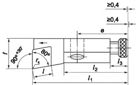
а) Для резцов-вставок высотой h_1 = 6 и 8 мм
