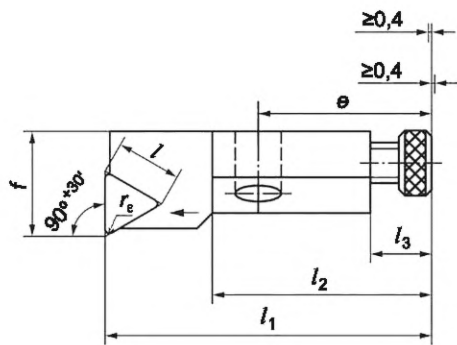
б) Для резцов-вставок высотой h_1 = 8, 10, 12, 16 и 20 мм
