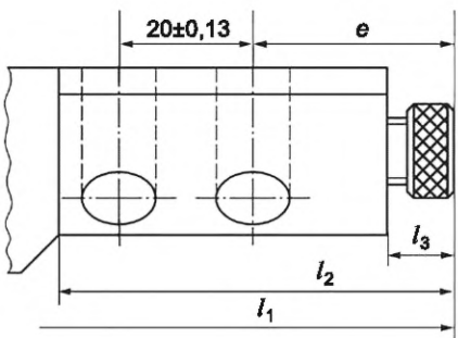
в) Для резцов-вставок высотой h_1 = 25 мм
