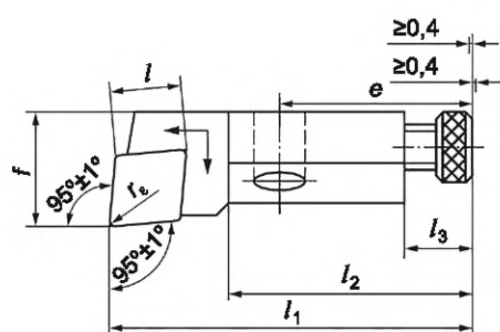
а) Для резцов-вставок высотой h_1 = 6, 8, 10, 12, 16 и 20 мм
