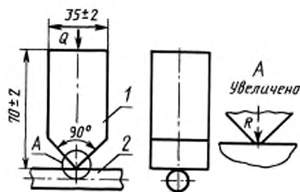
1 — угольник; 2 — образец кабеля; Q — нагрузка
