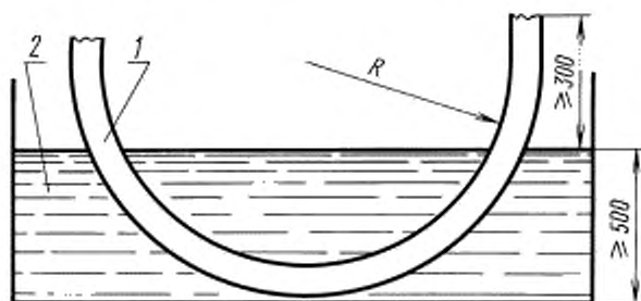
R — радиус изгиба; 1 — образец кабеля; 2 — соляная ванна
