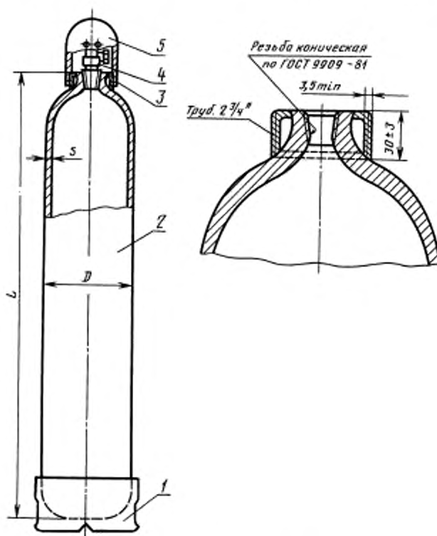
Горловина баллона
