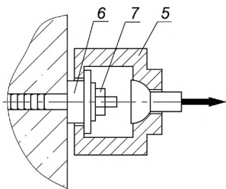
б) Приспособление для захвата механического, пластикового или клевого анкера
