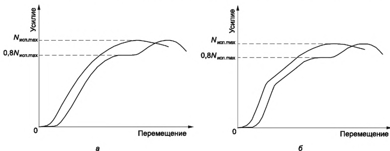
Рисунок 2 — Кривые нормального разрушения анкерного крепления без перегиба (а) и с перегибом (б) в интервале до 0,8N_{исп.max}
