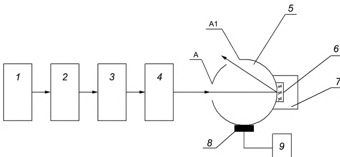
1 — лазер; 2 — модулятор; 3 — оптическая система; 4 — ослабитель (нейтральный светофильтр); 5 — фотометрический шар; 6 — зеркало (мера диффузного отражения); 7 — держатель оптики; 8 — измерительный преобразователь; 9 — регистрирующий прибор; А — входное окно фотометрического шара; А1 — выходное окно фотометрического шара
