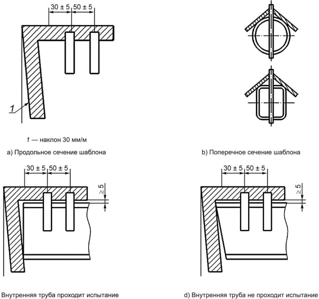
Рисунок 7 — Проверка прямоугольности концов внутренних труб
