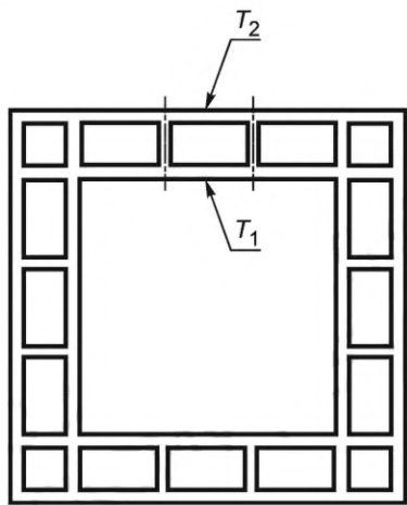
T_1, T_2 — внутренняя температура поверхности полости трубы Рисунок В.1 — Граничные условия
