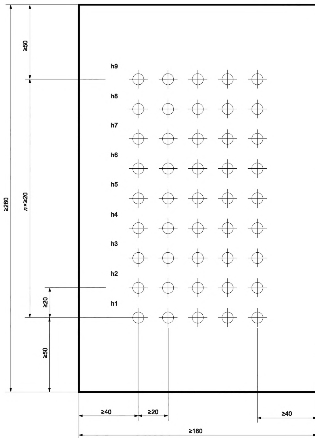
Рисунок 5 — Расположение ударов на одном испытуемом образце
