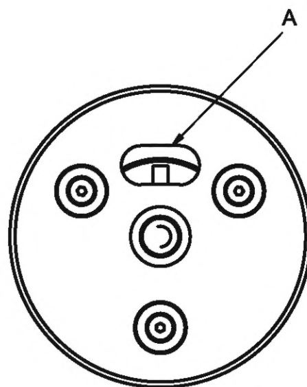
Рисунок 2 — Стальное основание с маркировочным отверстием
