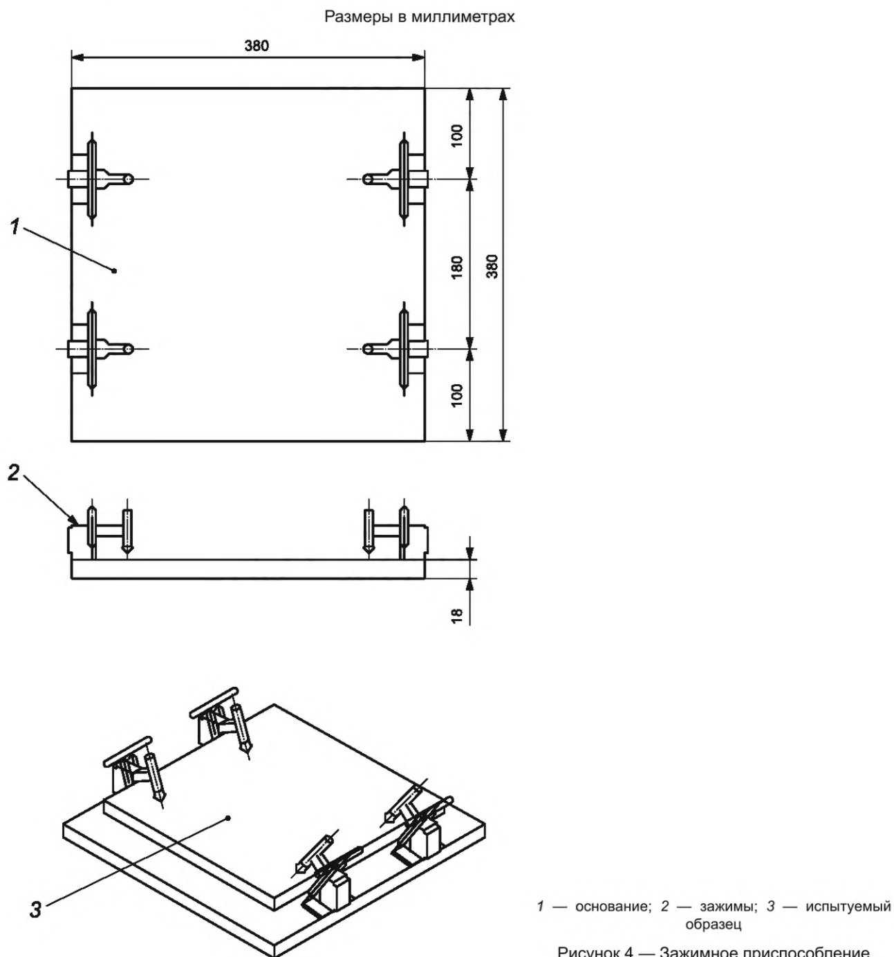
Рисунок 4 — Зажимное приспособление
