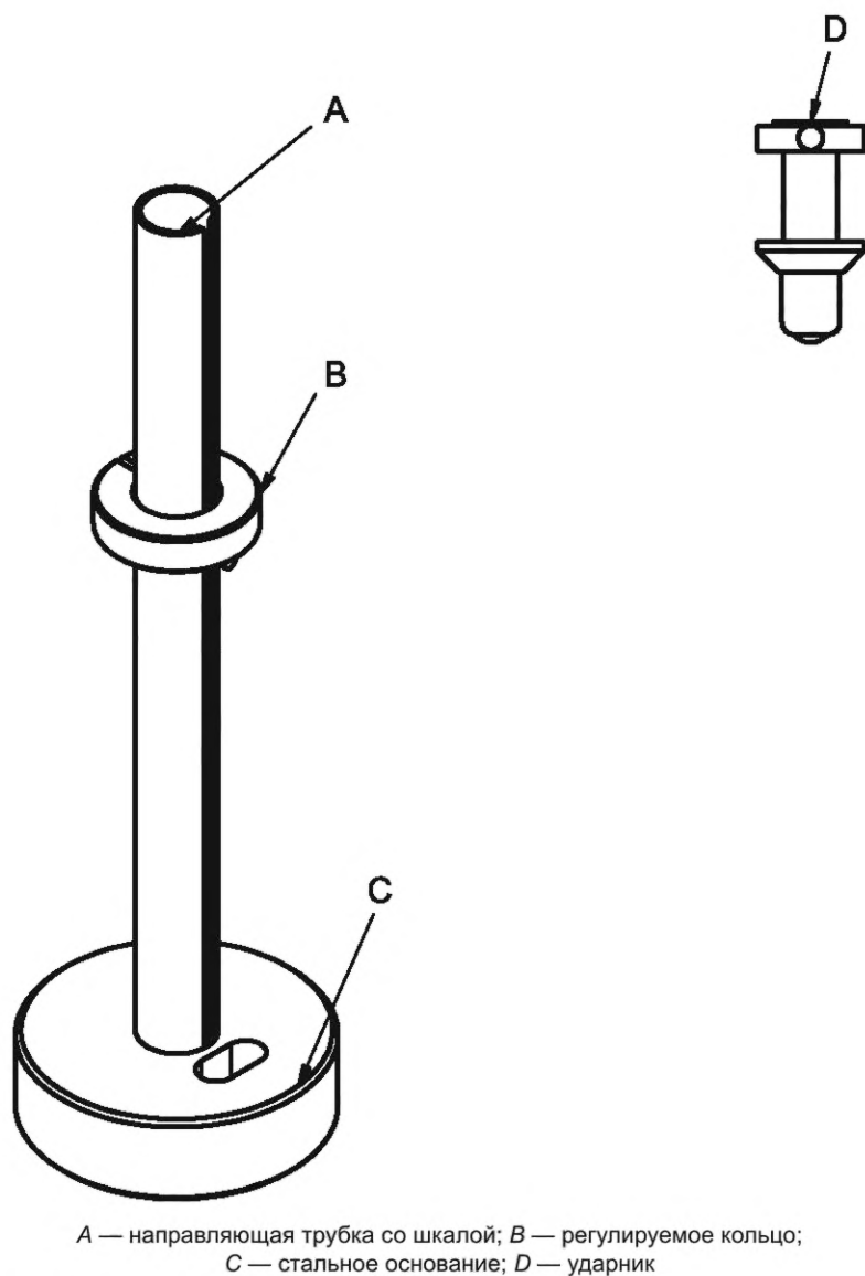
Рисунок 1 — Пример подходящей конфигурации средств испытаний
