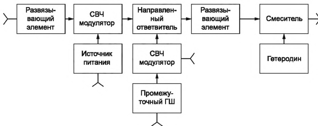
Рисунок А.1 — Возможный вариант структурной схемы преобразователя частоты
