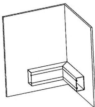
д) расположение для внутреннего угла без фасонной секции
