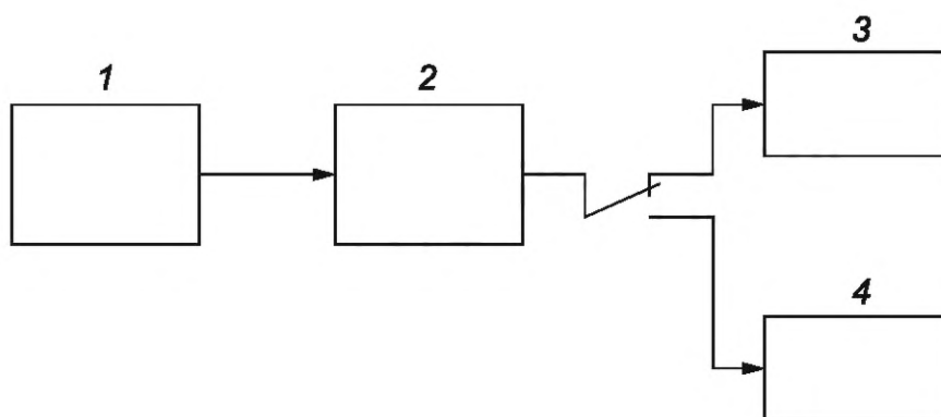
1 — осветитель и оптическая система; 2 — диссектор; 3 — осциллограф выделения строки (ОВС); 4 — измеритель постоянного тока
